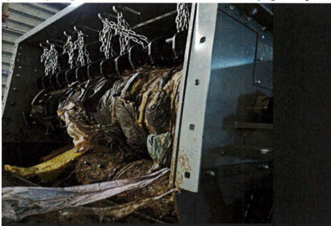
30 pav. Maišelių su atliekomis plėšimo įrenginys
