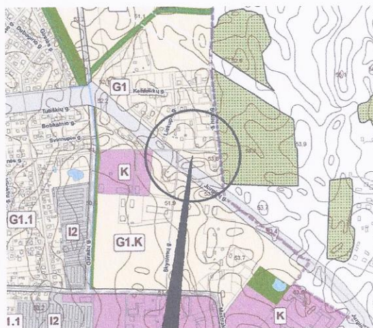
3.1.1. pav. Situacijos schema ( Panevėžio m. BP).
