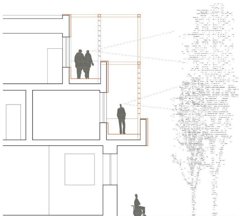
6 pav. Balkonų uždengimo principinė pjūvio schema
