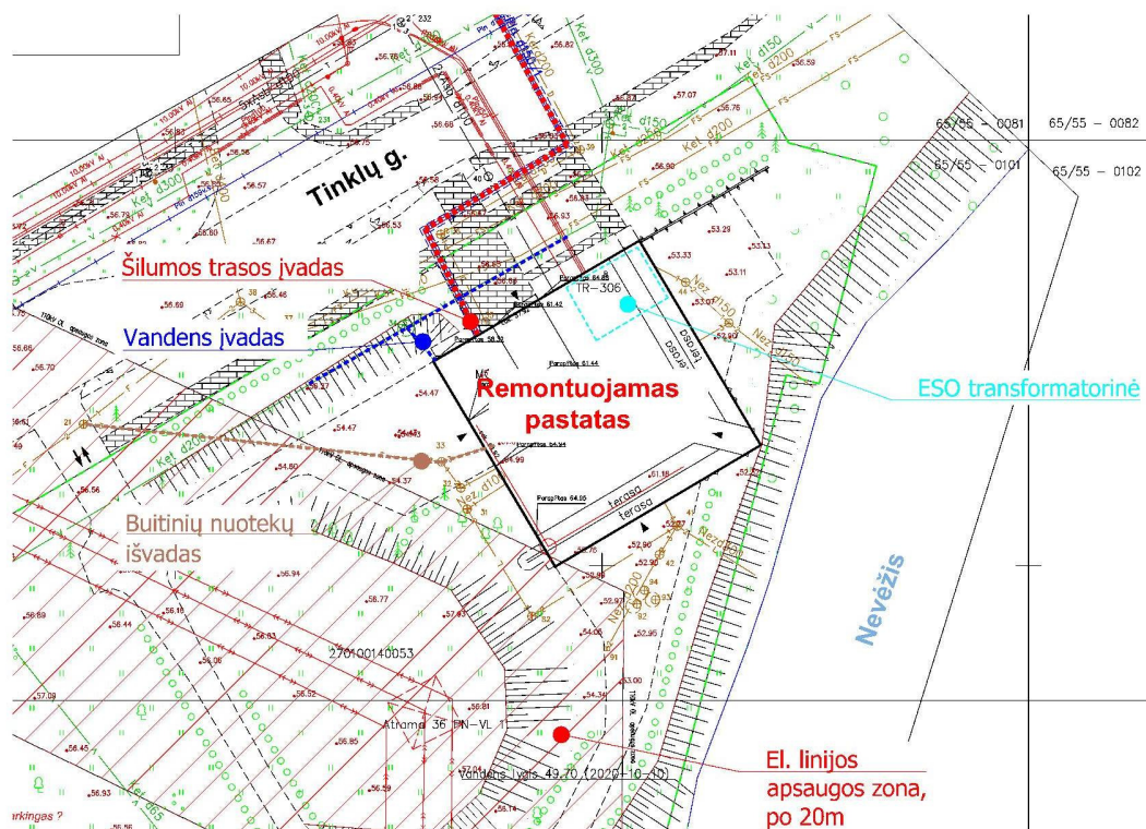
14 pav. Esamų įvadinių tinklų schema
