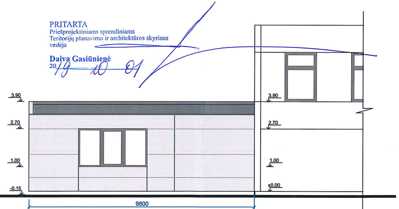
ŠIAURĖS VAKARŲ FASADAS M 1:100
