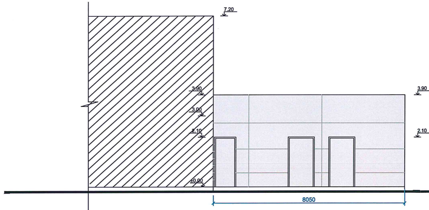
ŠIAURĖS RYTŲ FASADAS M 1:100
