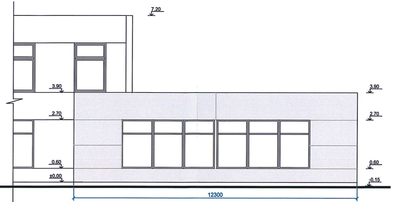
ŠIAURĖS VAKARŲ FASADAS M 1:100
