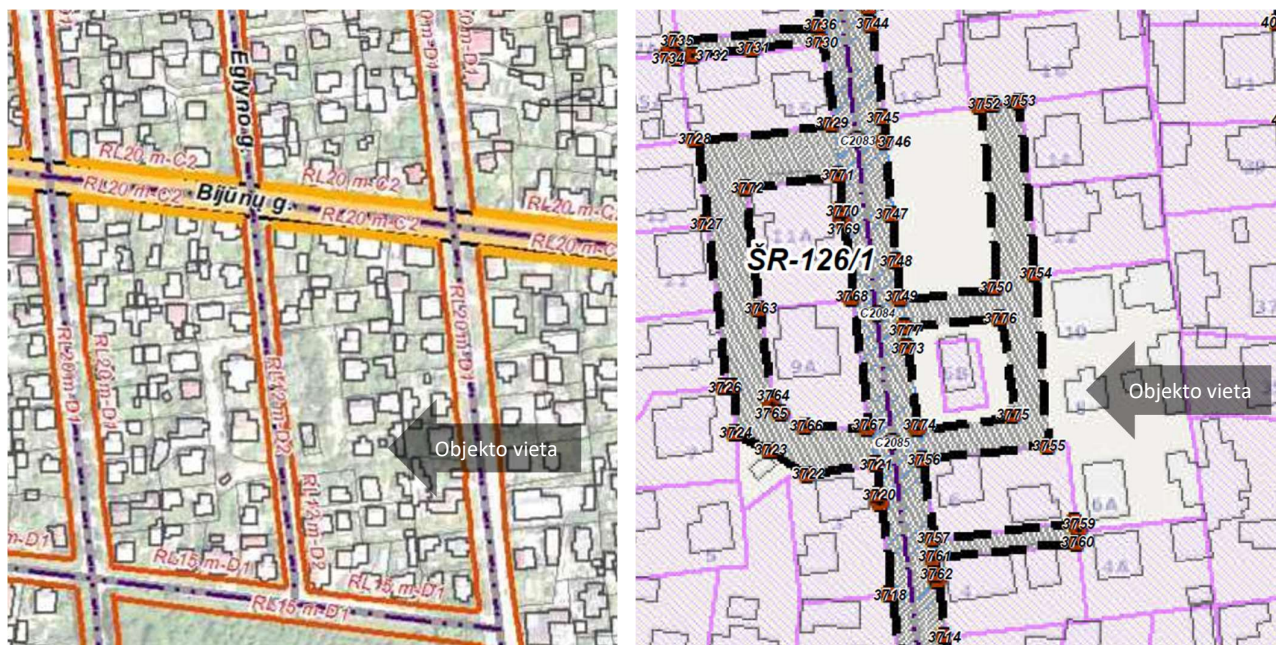
4 pav. Ištraukos iš Panevėžio miesto (šiaurinės dalies) susisiekimo komunikacijų specialiojo plano brėžinių
