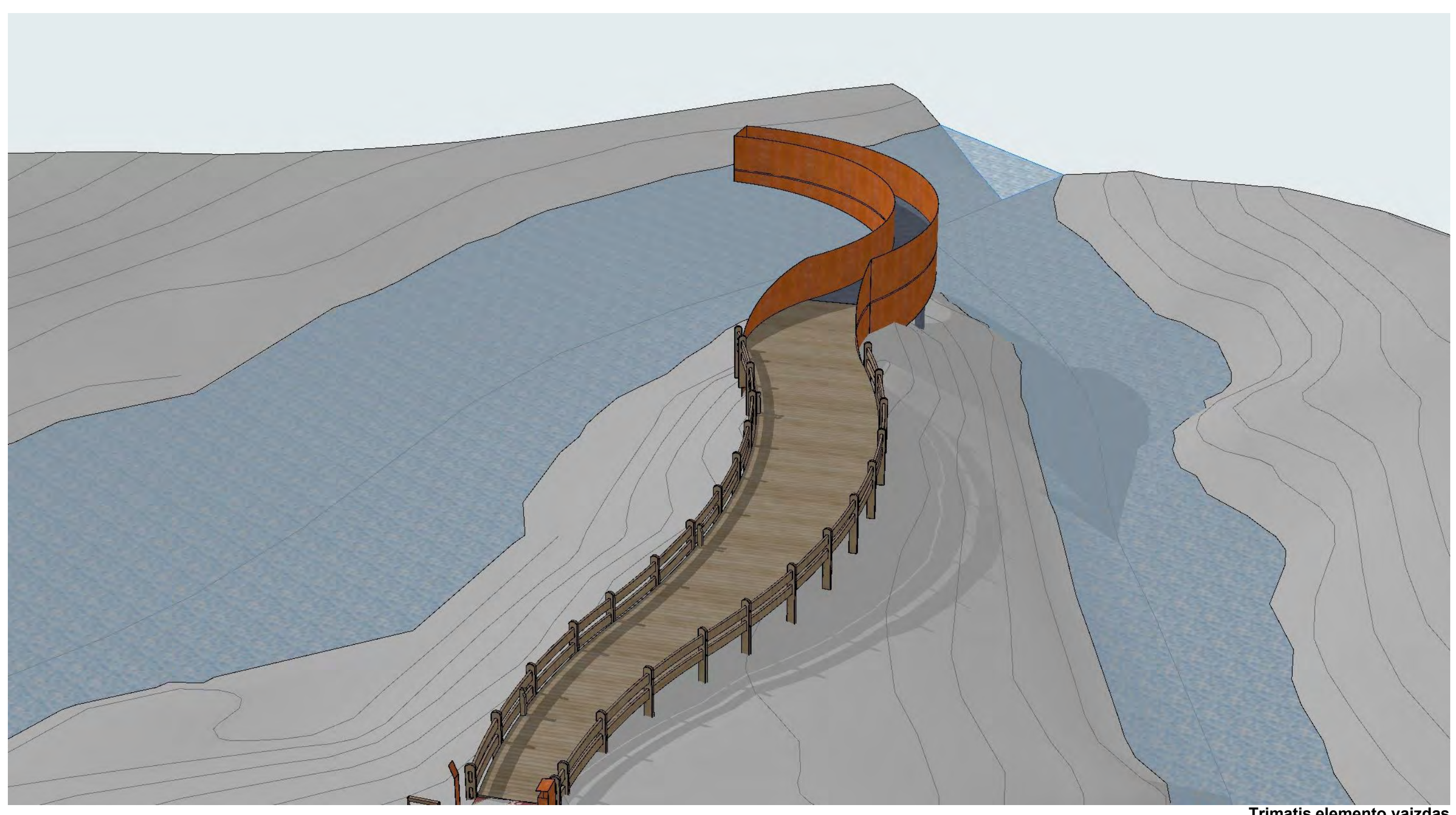
Trimatis elemento vaizdas
