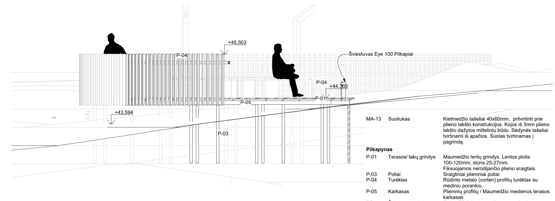
PT Terasos pilkapyne skersinis pjūvis S-P.1 1:50
