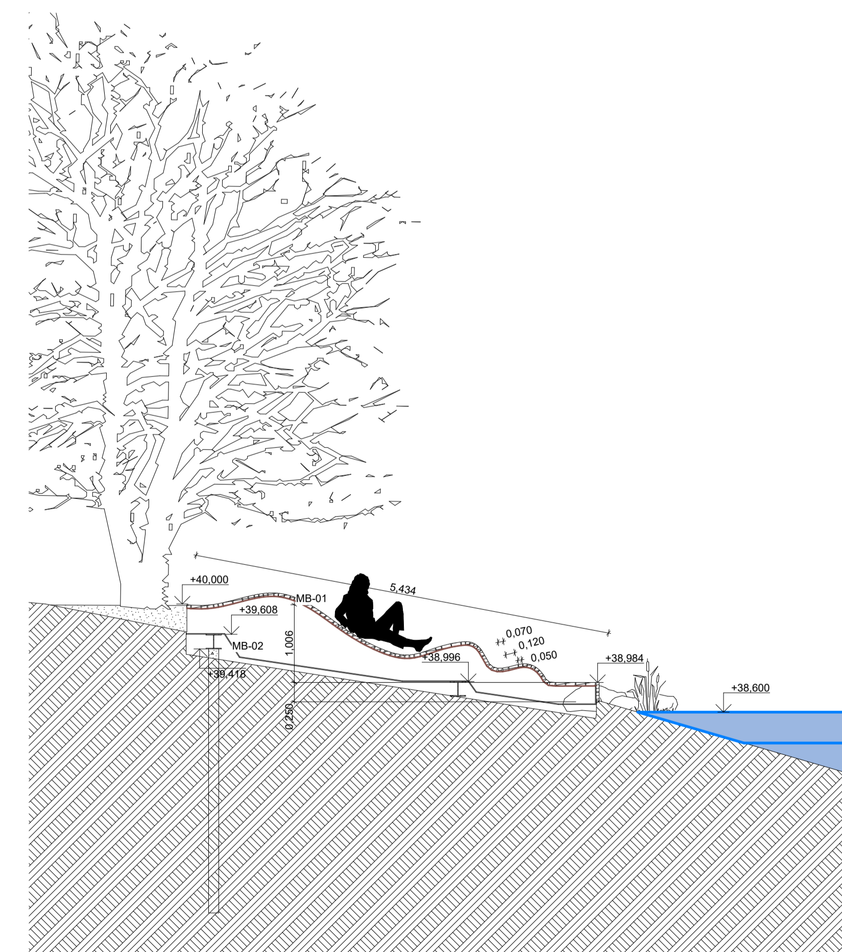
Maudyklos suolo/gulto skersinis pjūvis
