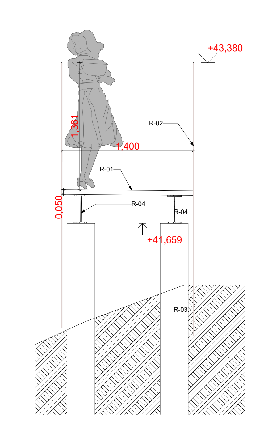
S-17 Skersinis pjūvis 1:25
