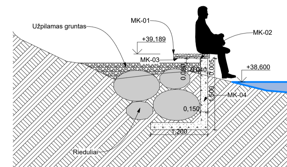
Krantinės skersinis pjūvis
