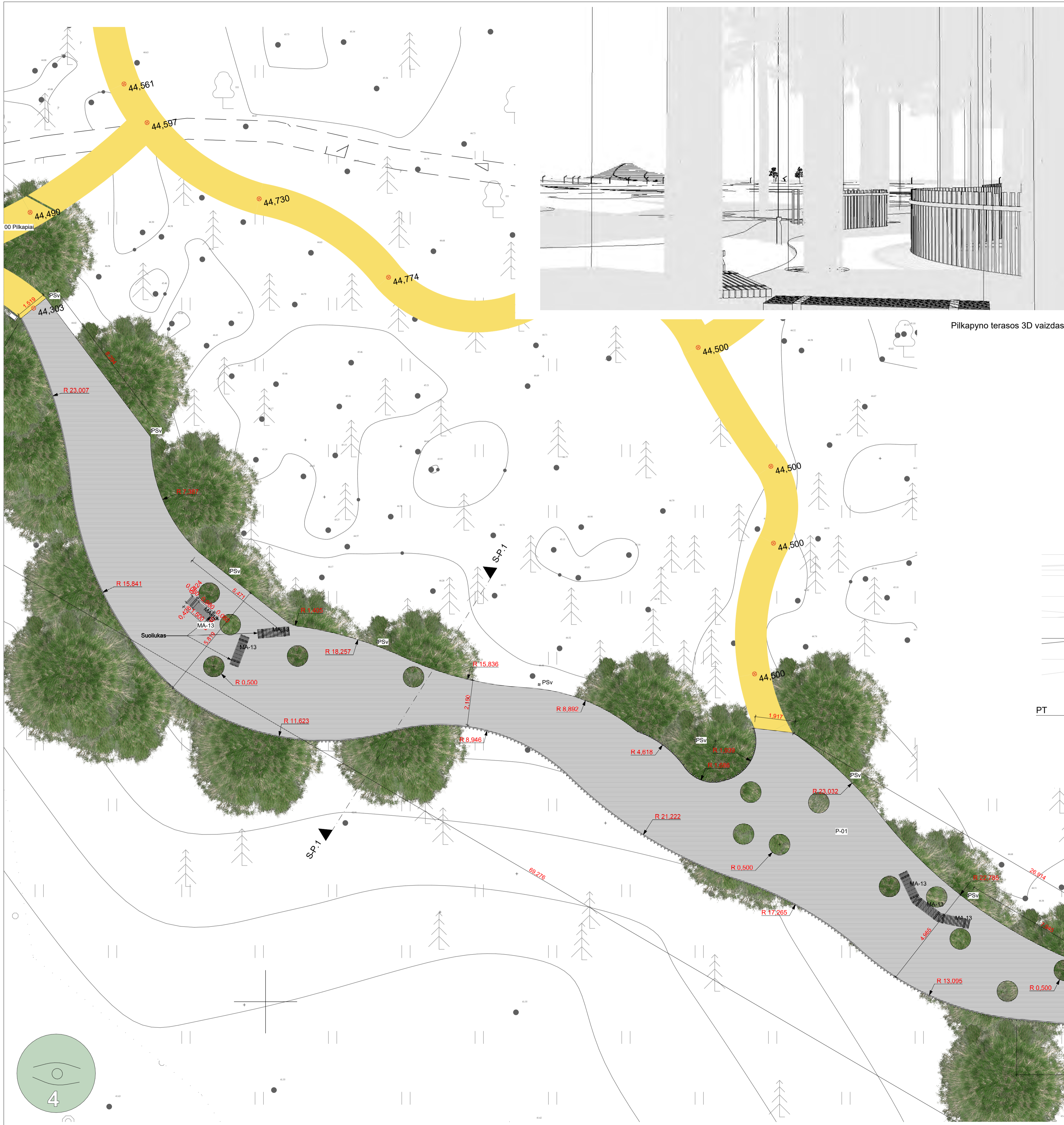
PT Terasos pilkapyne planas 1:100
