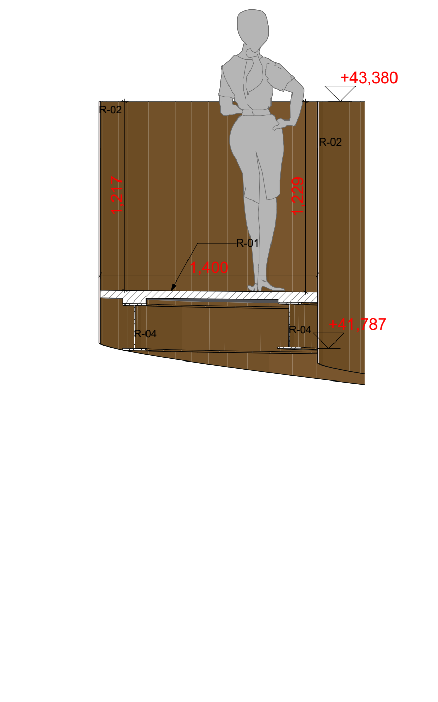
S-20 Skersinis pjūvis 1:25
