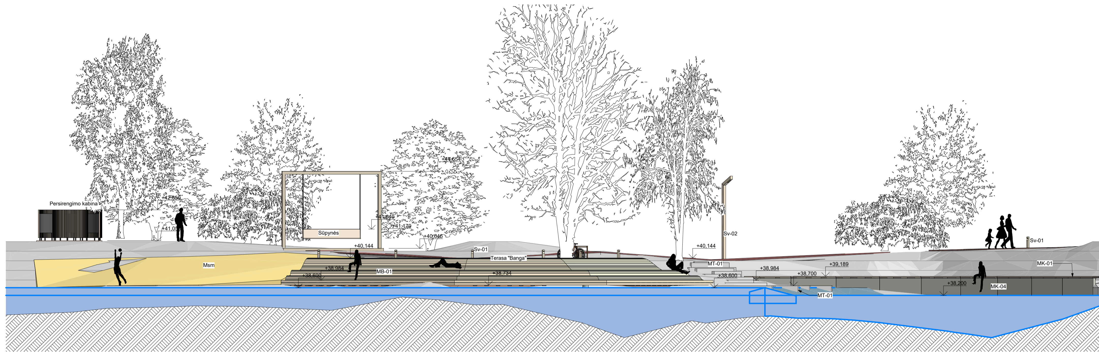
Išilginis maudyklos pjūvis nuo upės
