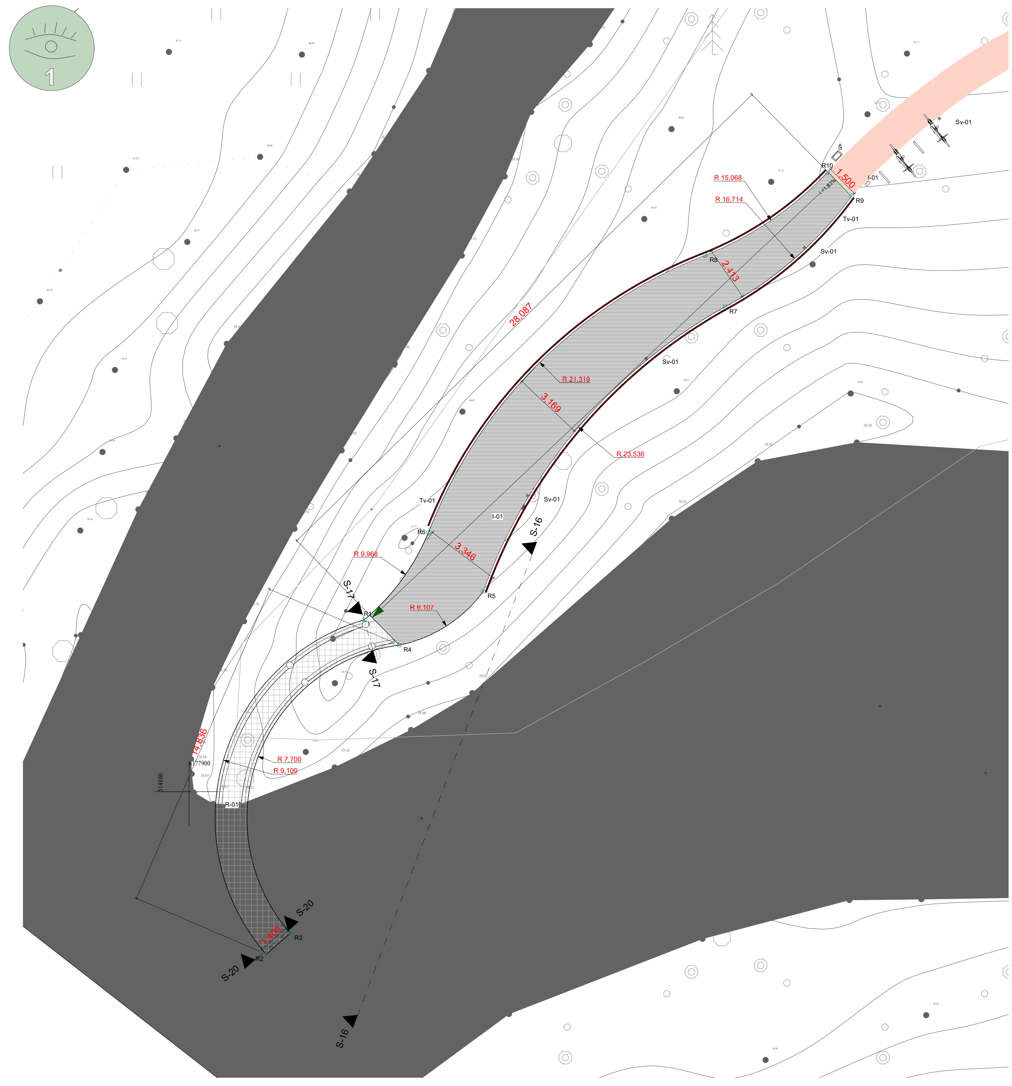
STE Santakos elemento - Rago planas 1:100
