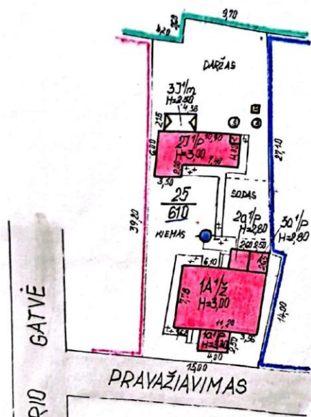
6 pav. ištrauka iš 1989 m statinių inventorinio plano
